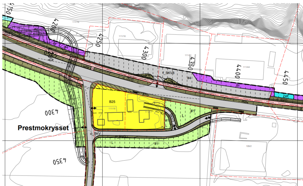
Figur 2 viser vedtatt reguleringsplan for området, 1-280 E14 Stjørådal-Hegramo, Gang- og sykkelveg.
